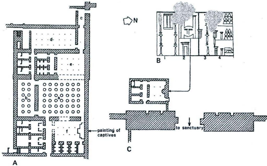
Reconstrucción. A: casa del rey; B: representación de la tumba de Meryra; C: parte del pequeño templo (Kemp 1976: 85, fig. 2)
